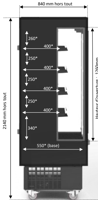
*Dimensions intérieures
