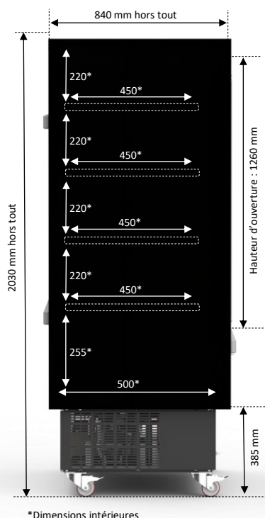
*Dimensions intérieures
