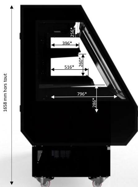
*Dimensions intérieures
